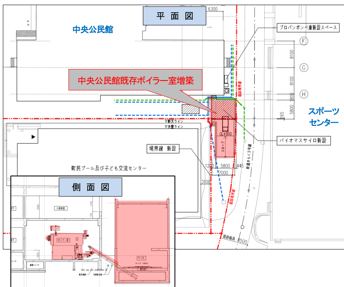
図 4.2.1.3 木質バイオマスボイラー導入箇所
